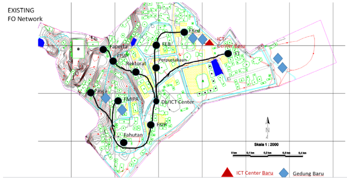
Gambar 5. Rencana Infrastruktur Jaringan Fiber Optik di Universitas Mulawarman
