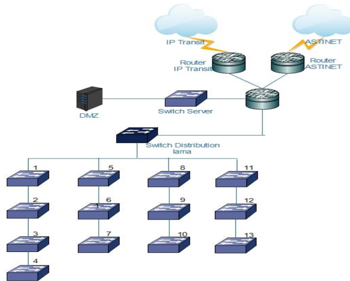
Gambar 4. Topologi Jaringan ke Fakultas Universitas Mulawarman
