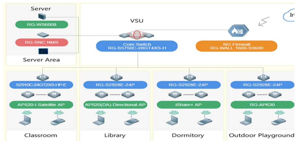
Gambar 10. Pengembangan Detail Infrastruktur Jaringan
