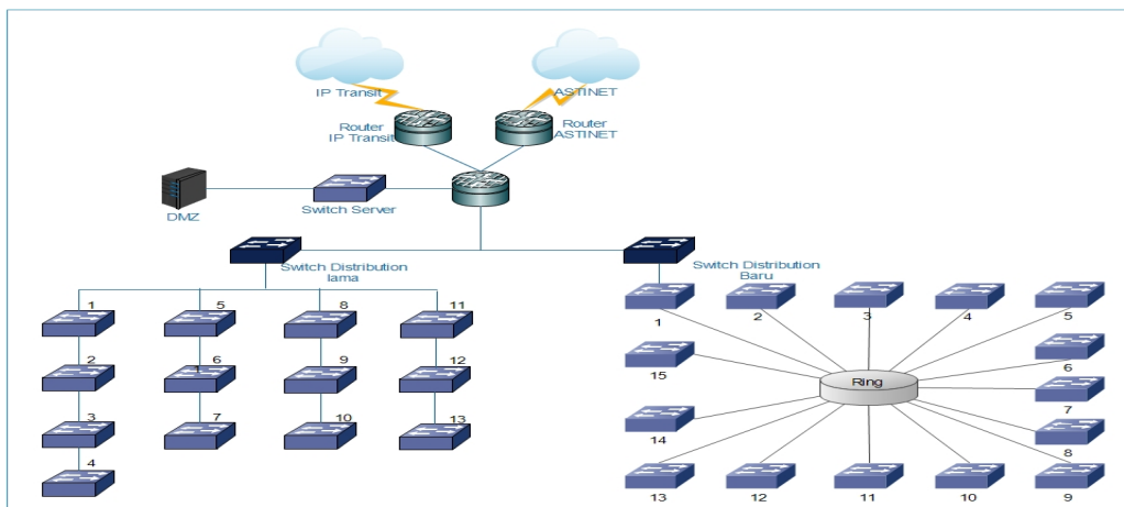
Gambar 7. Perencanaan Infrastruktur Jaringan Universitas Mulawarman
