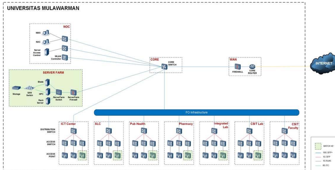
Gambar 8. Infrastruktur jaringan pada gedung baru (IDB)
