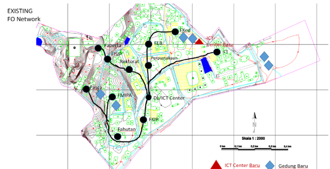
Gambar 6. Jaringan Fiber Optik di Universitas Mulawarman
